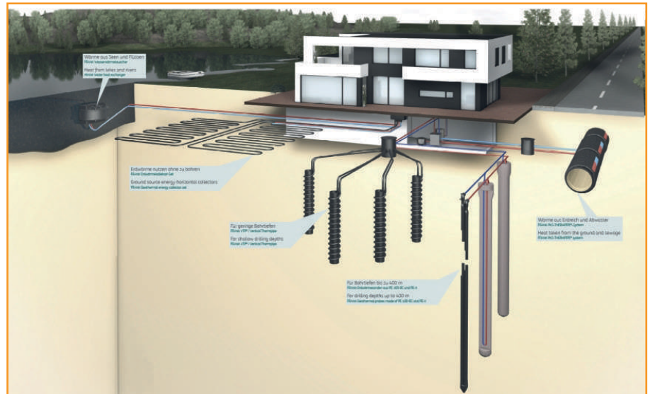
Alle Erdwärmesysteme aus dem Hause FRANK auf einem Blick.
